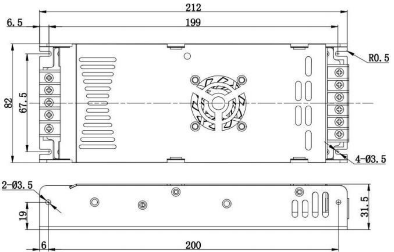
c. CL-AS5-300W-C 的外形尺寸
