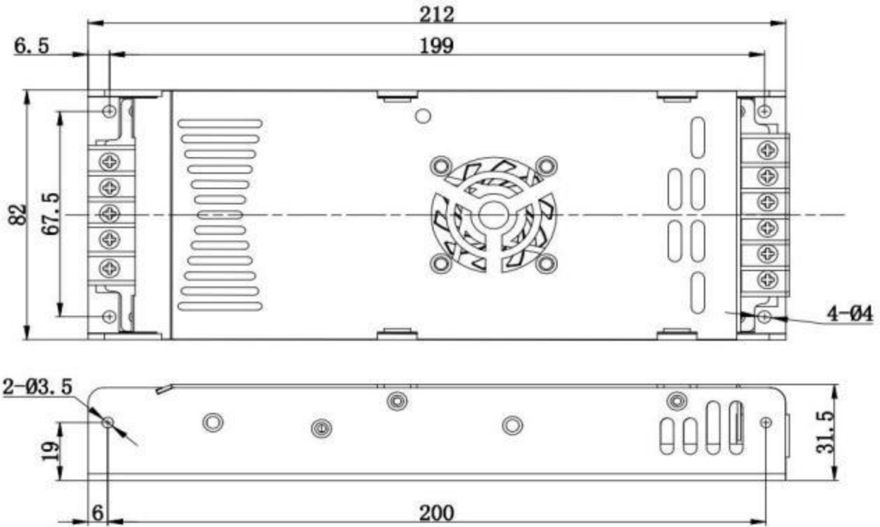
c. CL-AS5-300W-C 的外形尺寸
